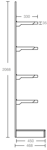
RETRO ESPOSITORE BACK DISPLAYER UNIT
