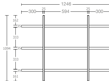
RETROALZATA BOTTIGLIERIA "TRALIX" P 270 "TRALIX" BOTTLE COMPARTMENT D 270
