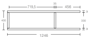
RETROALZATA BOTTIGLIERIA "CESAR" P 236 "CICLOPE" BOTTLE COMPARTMENT D 236
