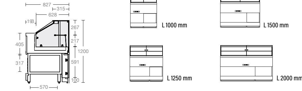
VETRINA REFRIGERATA STATICA CON MOTORE INCORPORATO H1200 P827 MM STATIC REFRIGERATED DISPLAY CASES WITH HERMETIC UNIT H1200 D827 MM
