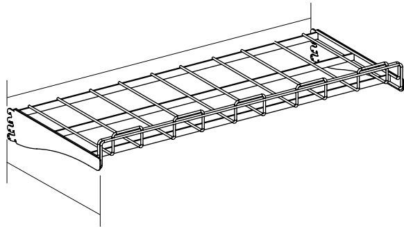
RIPIANO INCLINATO FRUTTA E VERDURA ZINCATO F&V GALVANIZED INCLINED SHELF L 1000 mm P 500 mm
