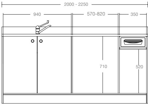
MODULO MACCHINA CAFFÈ RETRO COMBI CON 2 LAVELLI CAFFÈ MACHINE BACKCOUNTER COMBI WITH 2 SINK
