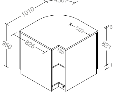
ANGOLO ESTERNO CURVO 90° L1010 H950 P1010 EXTERNAL CURVED CORNER 90° W1010 H950 P1010
