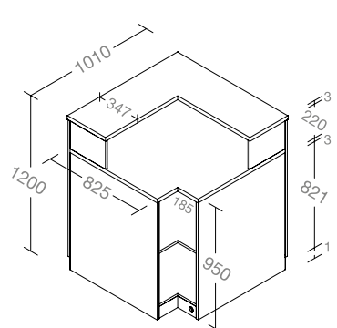
ANGOLO ESTERNO BAR 90° L1000 H1200 P1000 MM EXTERNAL BAR CORNER 90° W1000 H1200 D1000 MM
