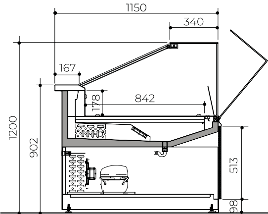
FREDDO VENTILATO _ COLD VENTILATED Dim: 1500-2000-2500-3000 mm
