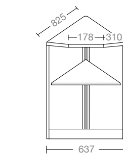
ANGOLO INTERNO 45° L795 H950 P825 MM INTERNAL CORNER 45° W795 H950 D825 MM
