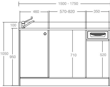
MODULO MACCHINA CAFFÈ RETRO COMBI CON 1 LAVELLO CAFFÈ MACHINE BACKCOUNTER COMBI WITH 1 SINK
