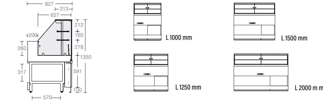
VETRINA REFRIGERATA STATICA CON MOTORE INCORPORATO H1350 D827 MM STATIC REFRIGERATED DISPLAY CASES WITH HERMETIC UNIT H1350 D827 MM
