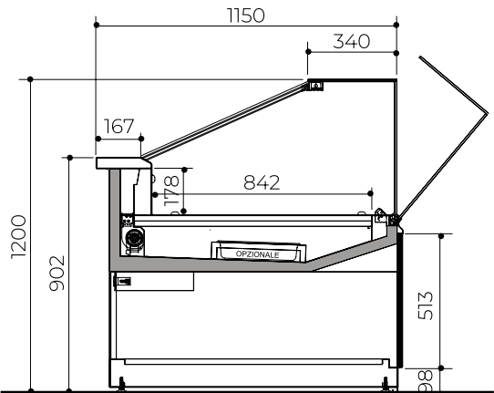
CALDO VENTILATO _ HOT VENTILATED Dim: 1500-2000-2500-3000 mm
