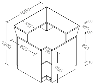
ANGOLO ESTERNO BAR 90° L1090 H1200 P1090 CON SOTTOBANCALINA IN METALLO EXTERNAL BAR CORNER 90° W1090 H1200 P1090 WITH STEEL UPPER TOP STRUCTURE
