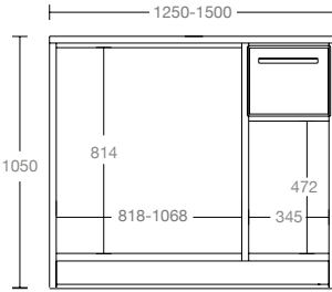
BASE PER MACCHINA CAFFÈ COFFEE MACHINE UNIT
