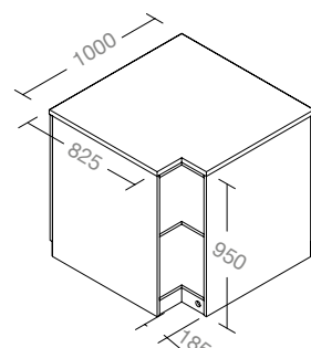
ANGOLO ESTERNO 90° L1000 H950 P1000 MM EXTERNAL CORNER 90° W1000 H950 D1000 MM
